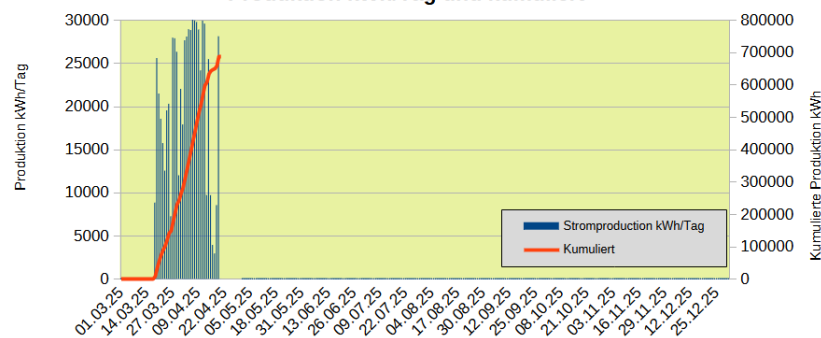
Produktion kWh/Tag und kumuliert
